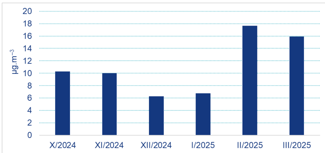
Obrázek 1 Průměrné měsíční koncentrace PM 10 , Jeseník-lázně, říjen 2024 až březen 2025
