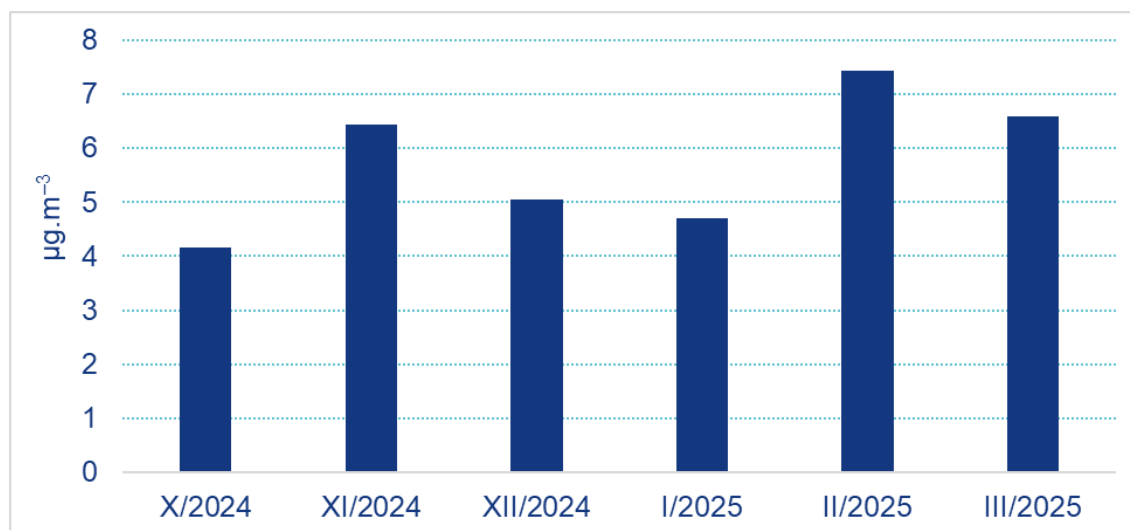
Obrázek 4 Průměrné měsíční koncentrace NO x , Jeseník-lázně, říjen 2024 až březen 2025
