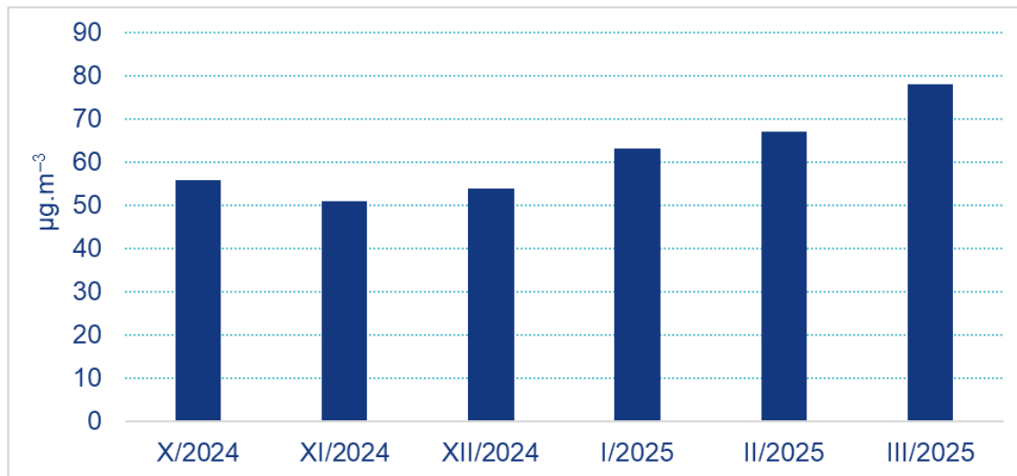
Obrázek 5 Průměrné měsíční koncentrace O_3 , Jeseník-lázně, říjen 2024 až březen 2025
