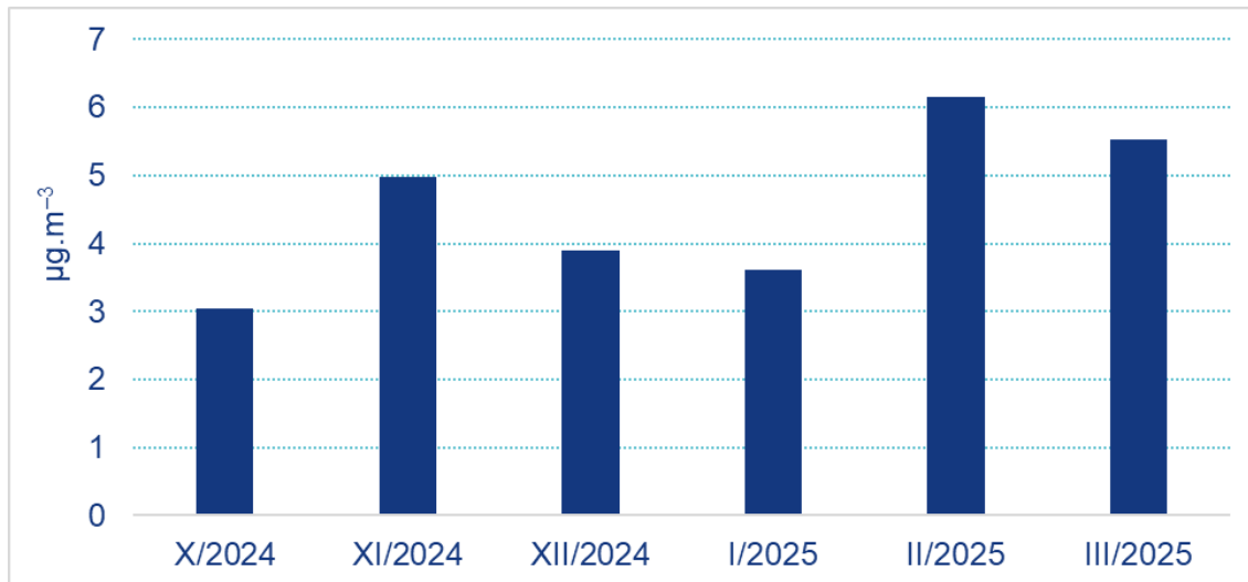
Obrázek 3 Průměrné měsíční koncentrace NO 2 , Jeseník-lázně, říjen 2024 až březen 2025
